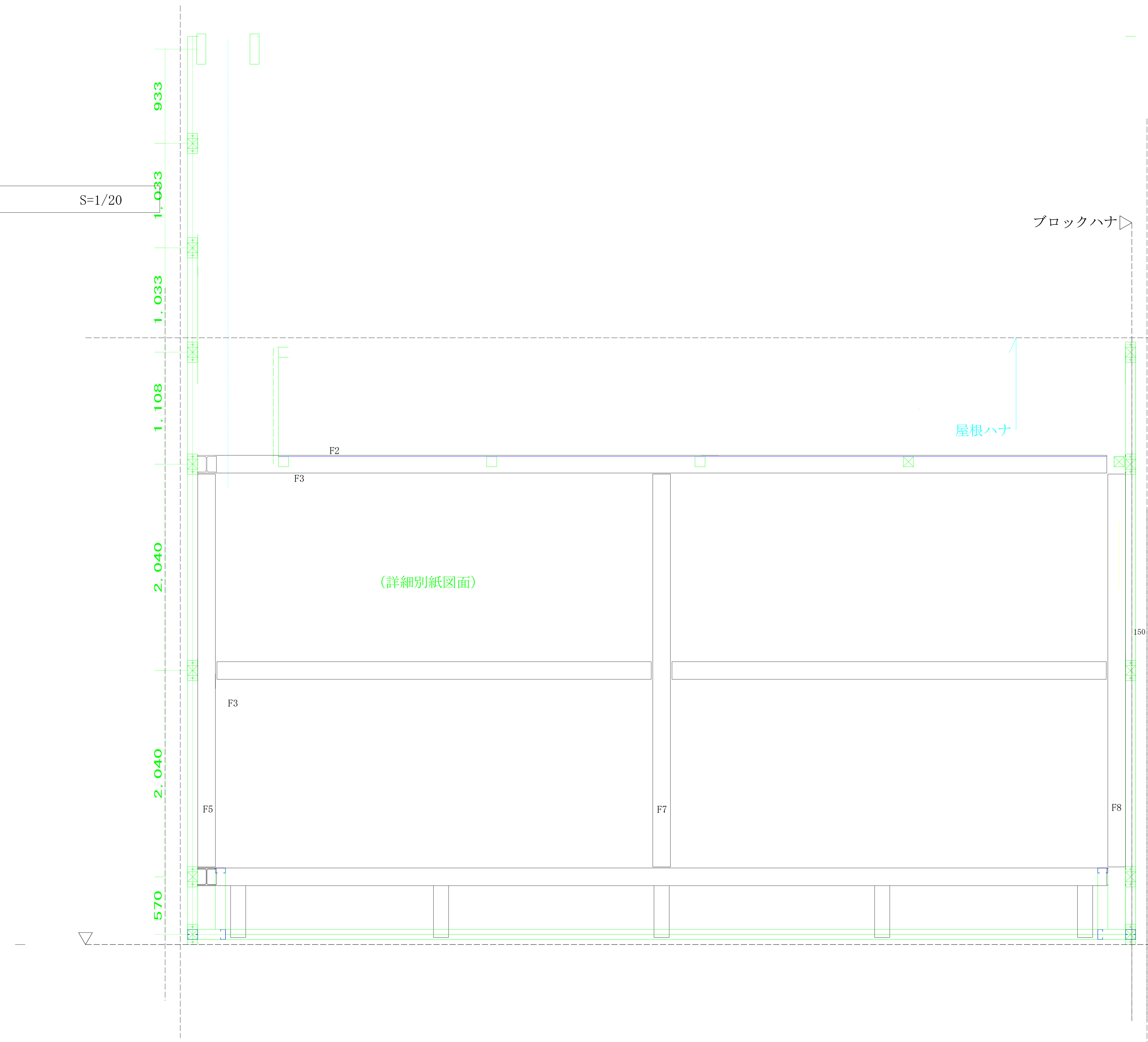
1通り側面 S=1/20
